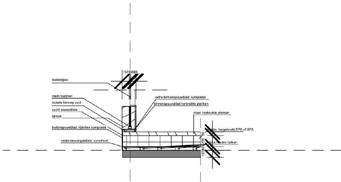
detail 3: vloer naar raam
