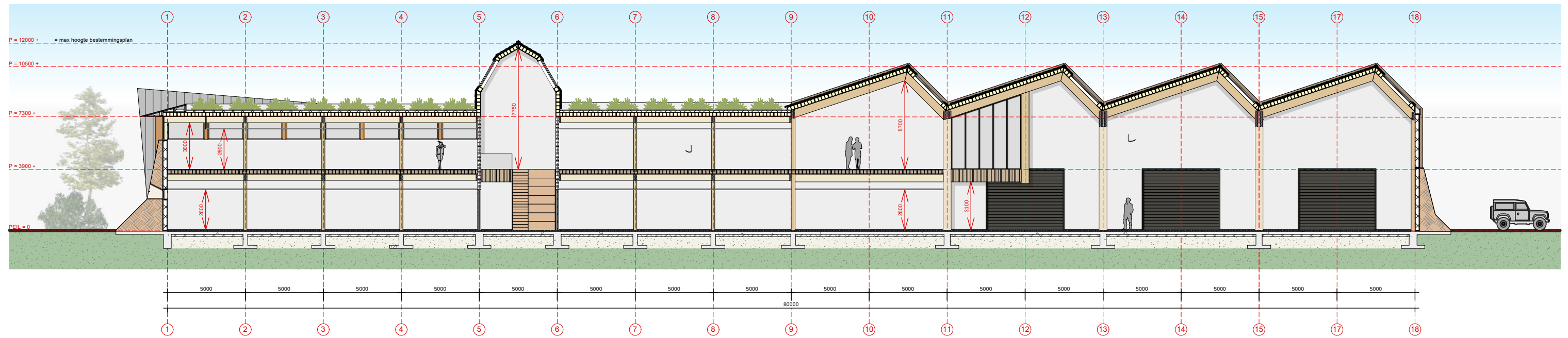
Doorsnede A-A
