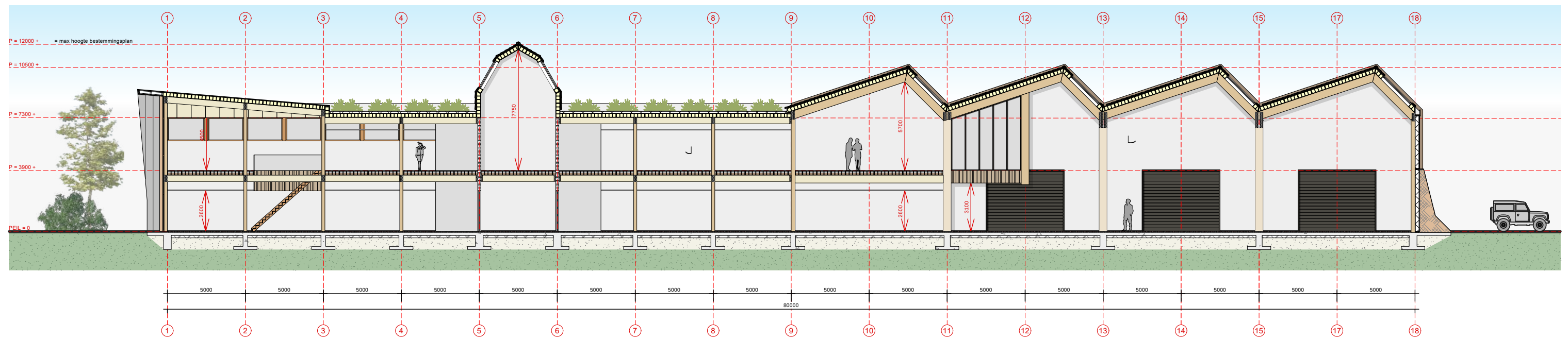
Doorsnede B-B
