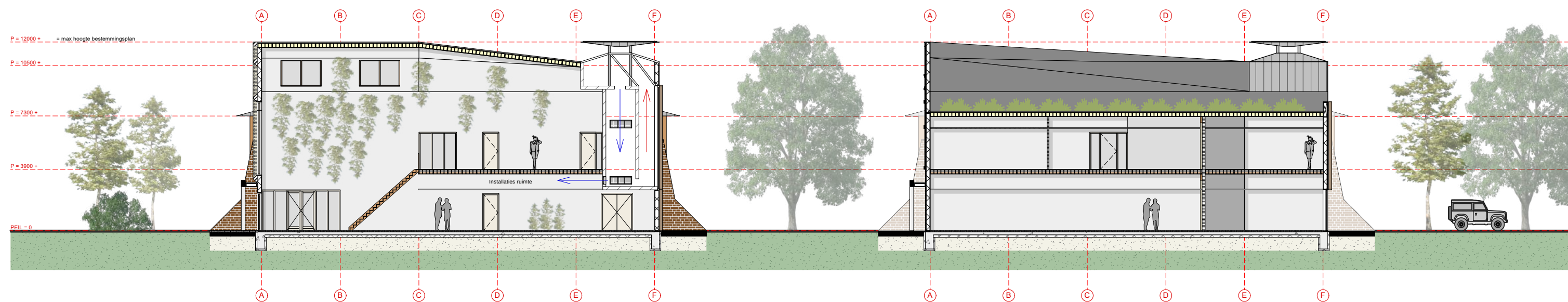
Doorsnede C-C
