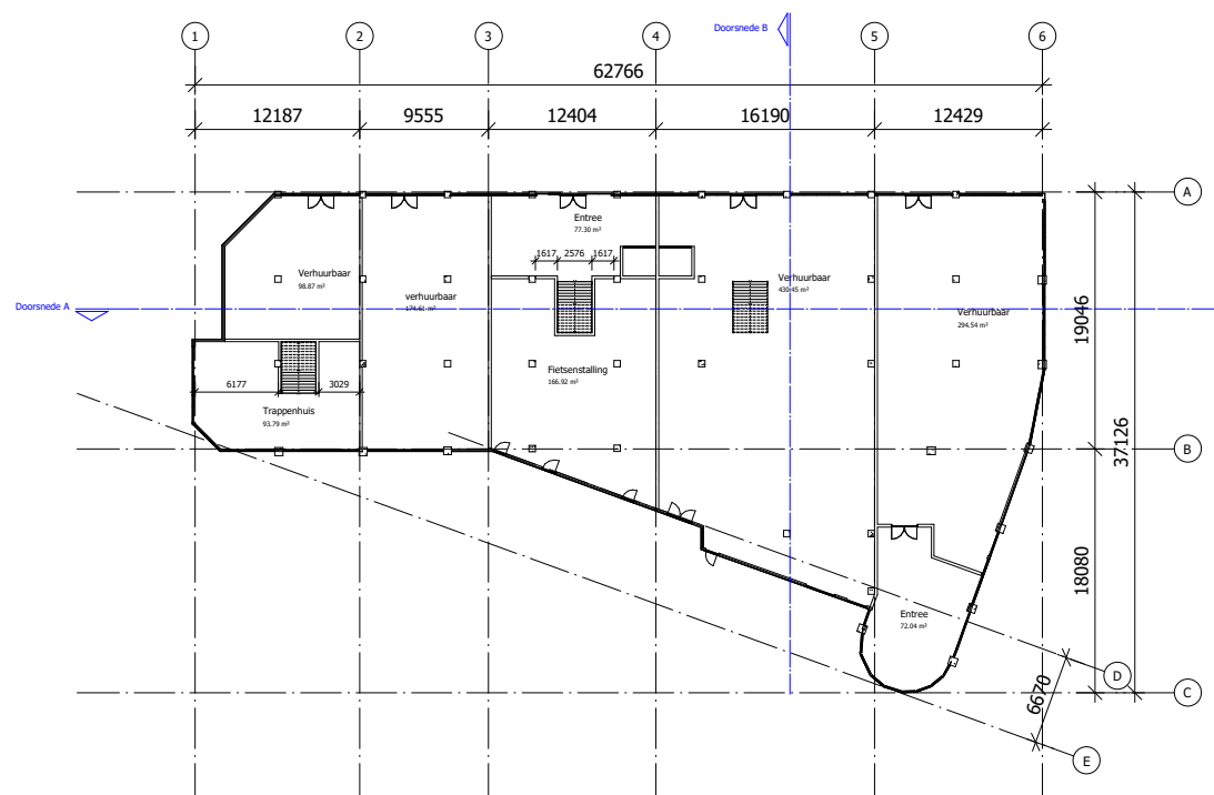
Begane grond nieuw
