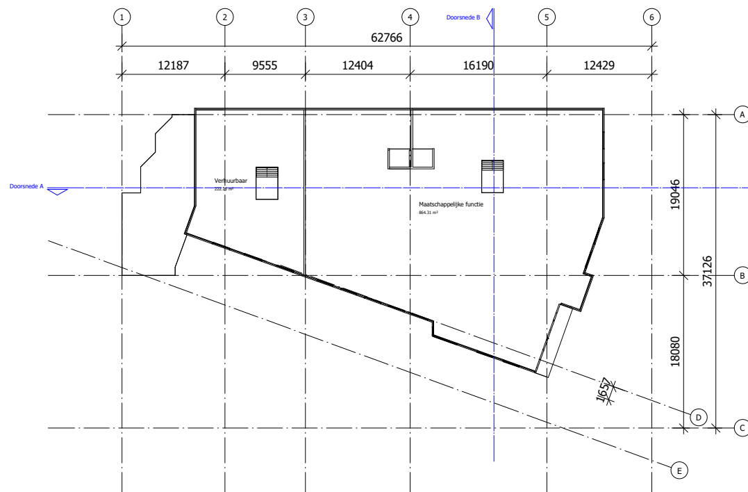
Tweede verdieping nieuw
