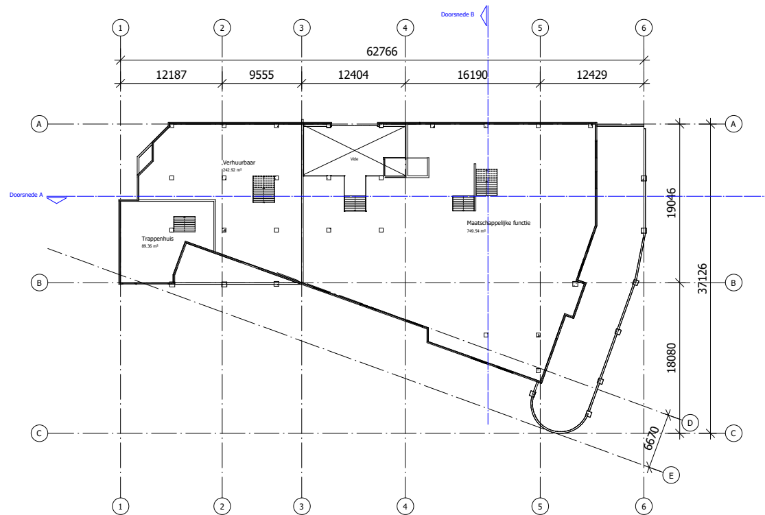
Eerste verdieping nieuw
