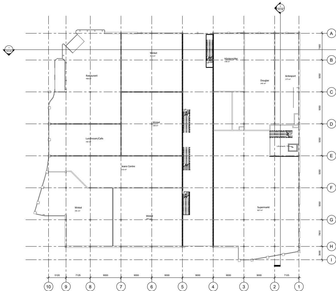
Begane grond nieuw
