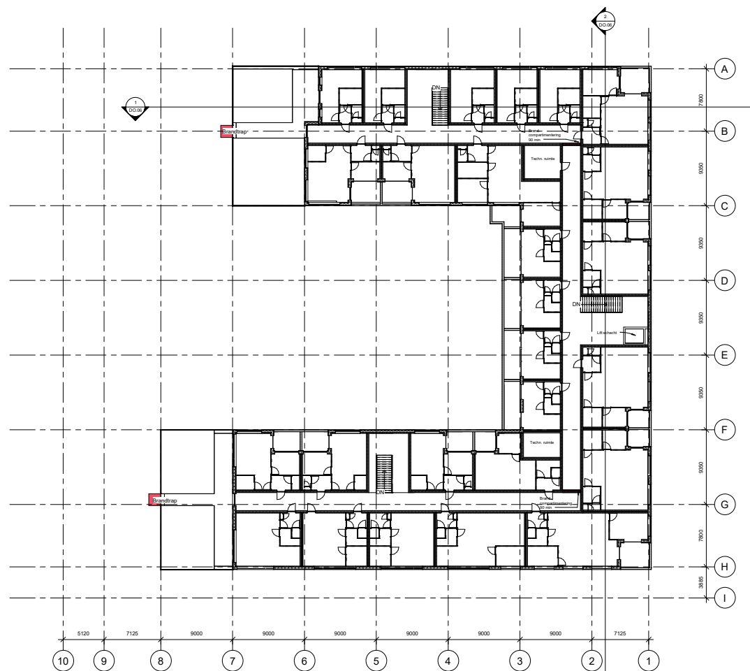
Tweede verdieping nieuw
